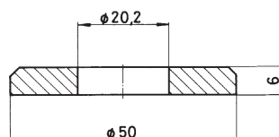
Deska k přírubě Objednávací číslo: LA 02.002
