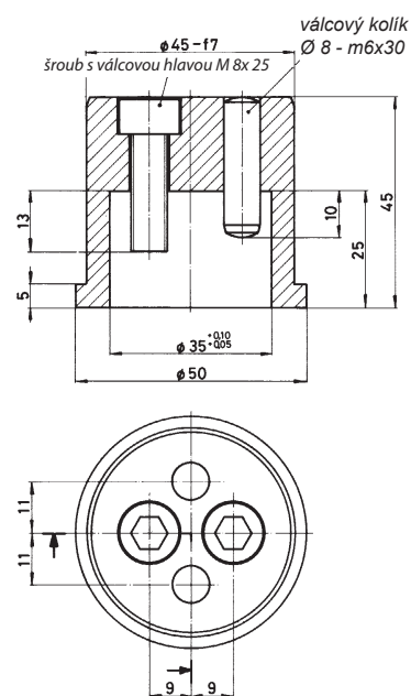
Příruba pro MD 51/180 B Objednávací číslo: LA 01.000
