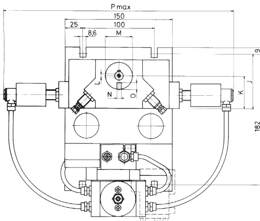
hnací hřídel MD 51/180 B
