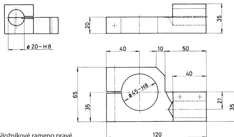
Výložníkové rameno pravé
