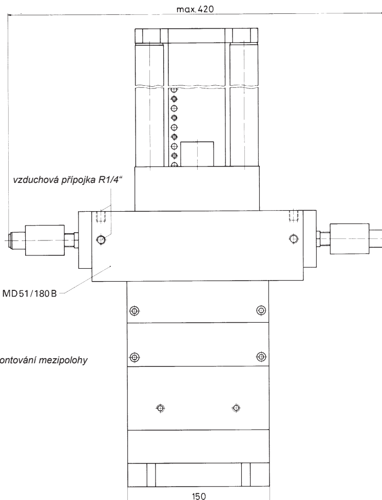
DL 51/200 s mezípolohou
