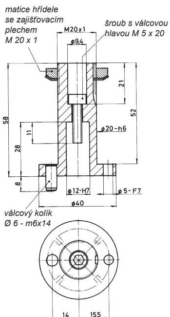
Příruba pro MD 32/180 B Objednávací číslo: LA 02.005
