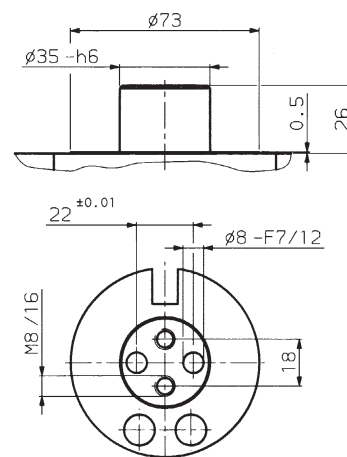
hnací hřídel MD 51/180 B
